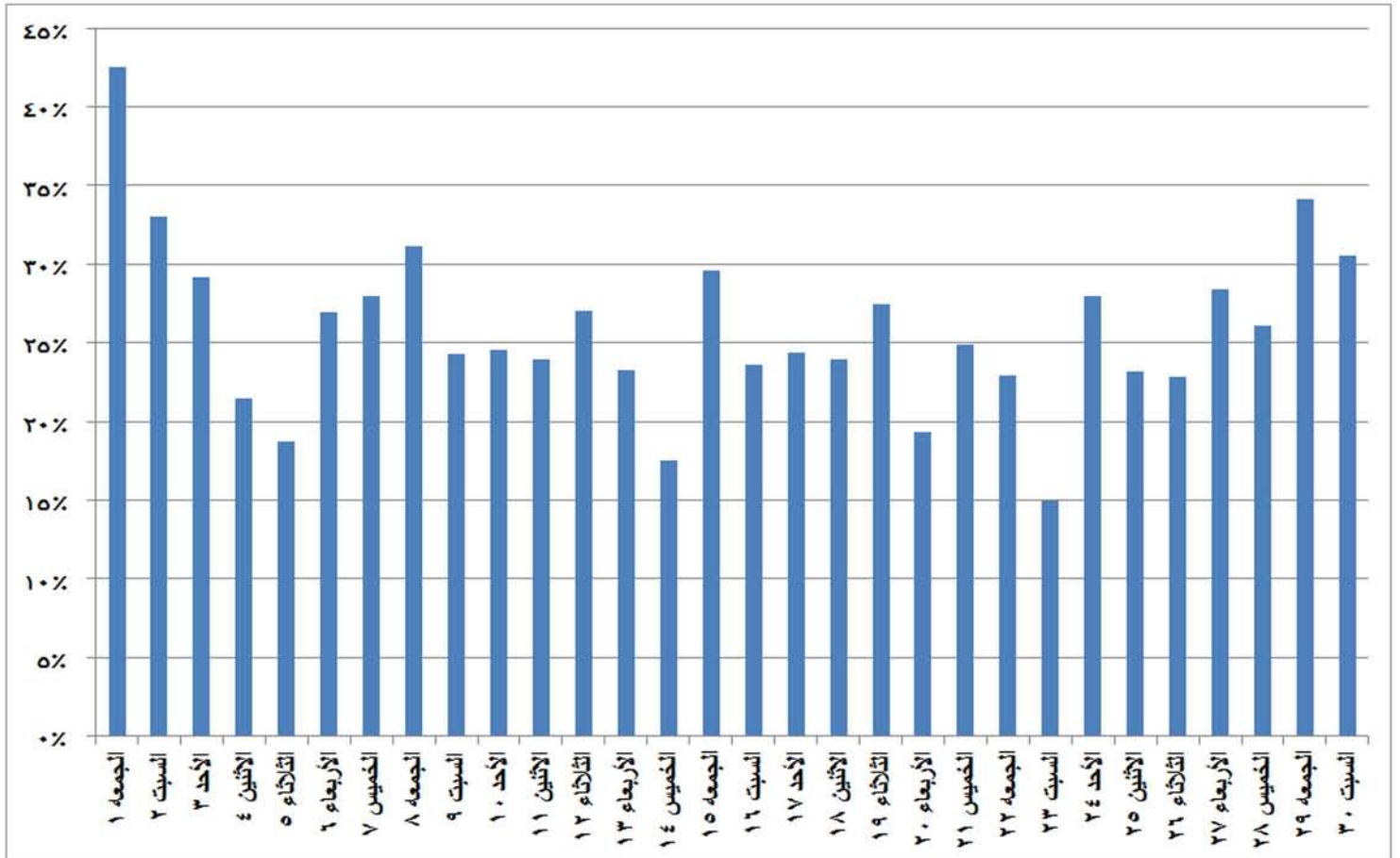
شكل (٢٨) نسب الفائض للحمل الاقصى المسجل يوميا خلال شهر سبتمبر ٢٠١٧
