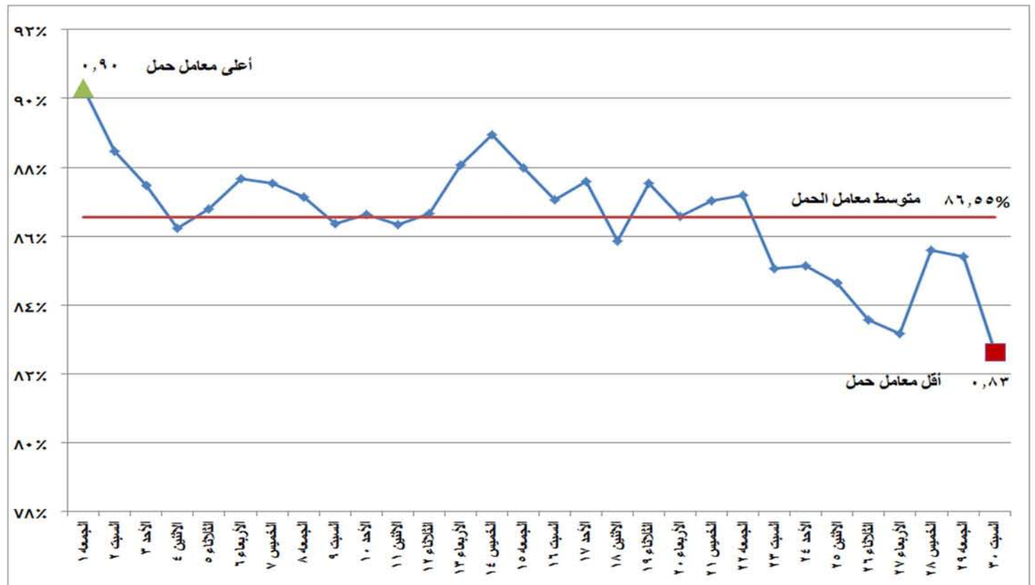
شكل (١٢) إجمالي معامل الحمل لوحدات الانتاج خلال شهر سبتمبر ٢٠١٧
