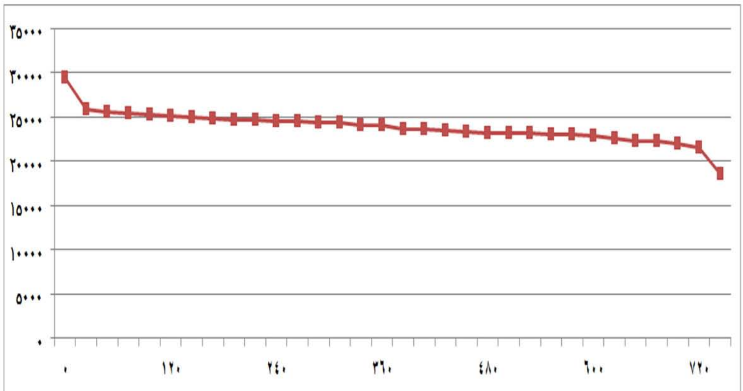
شكل (٨) المنحنى الشهري لفترة الحمل لشهر سبتمبر ٢٠١٧
