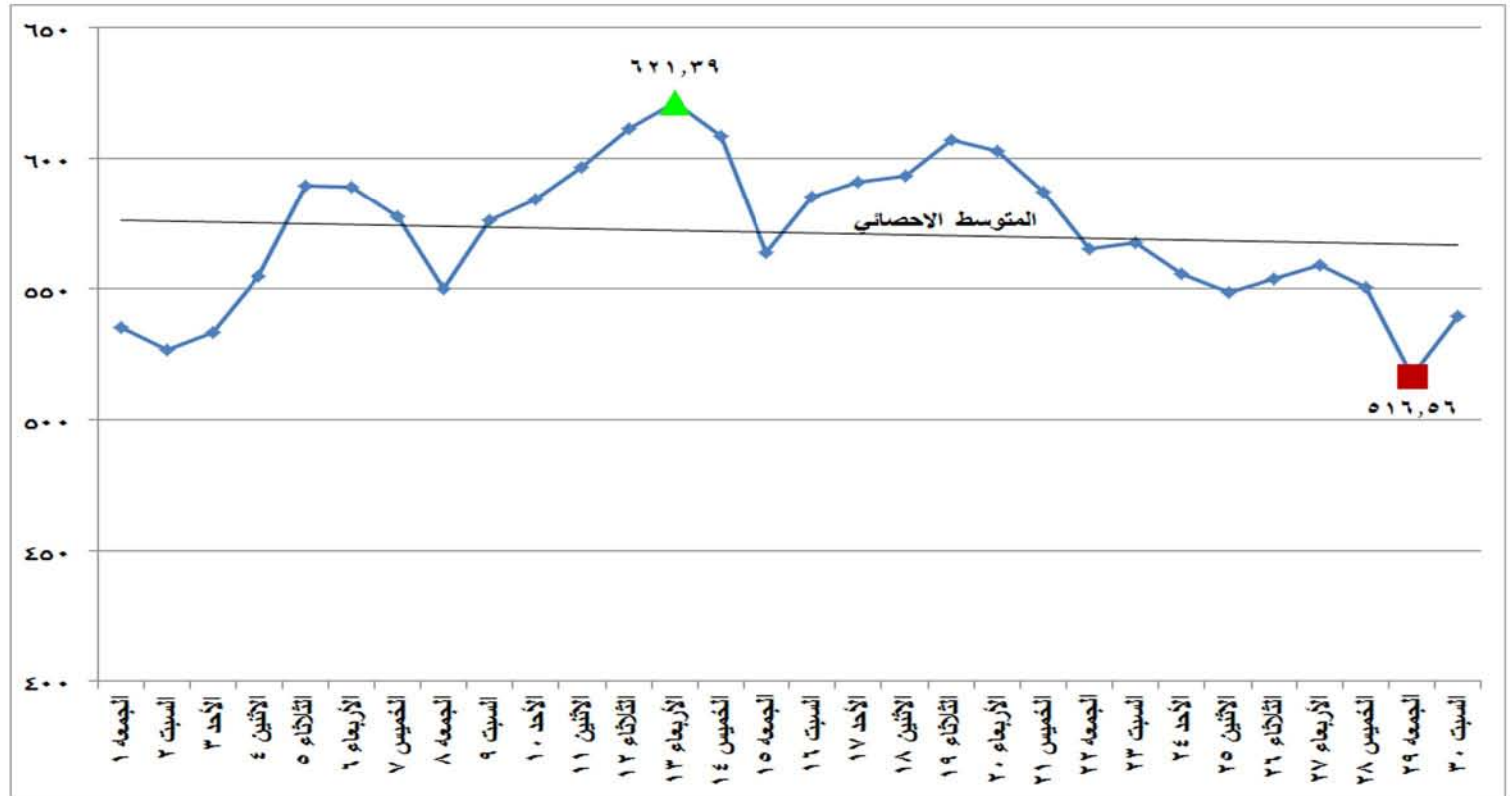
شكل (١٥) إجمالي الطاقة الكهربائية المنتجة من كل المصادر الأولية خلال شهر سبتمبر ٢٠١٧
