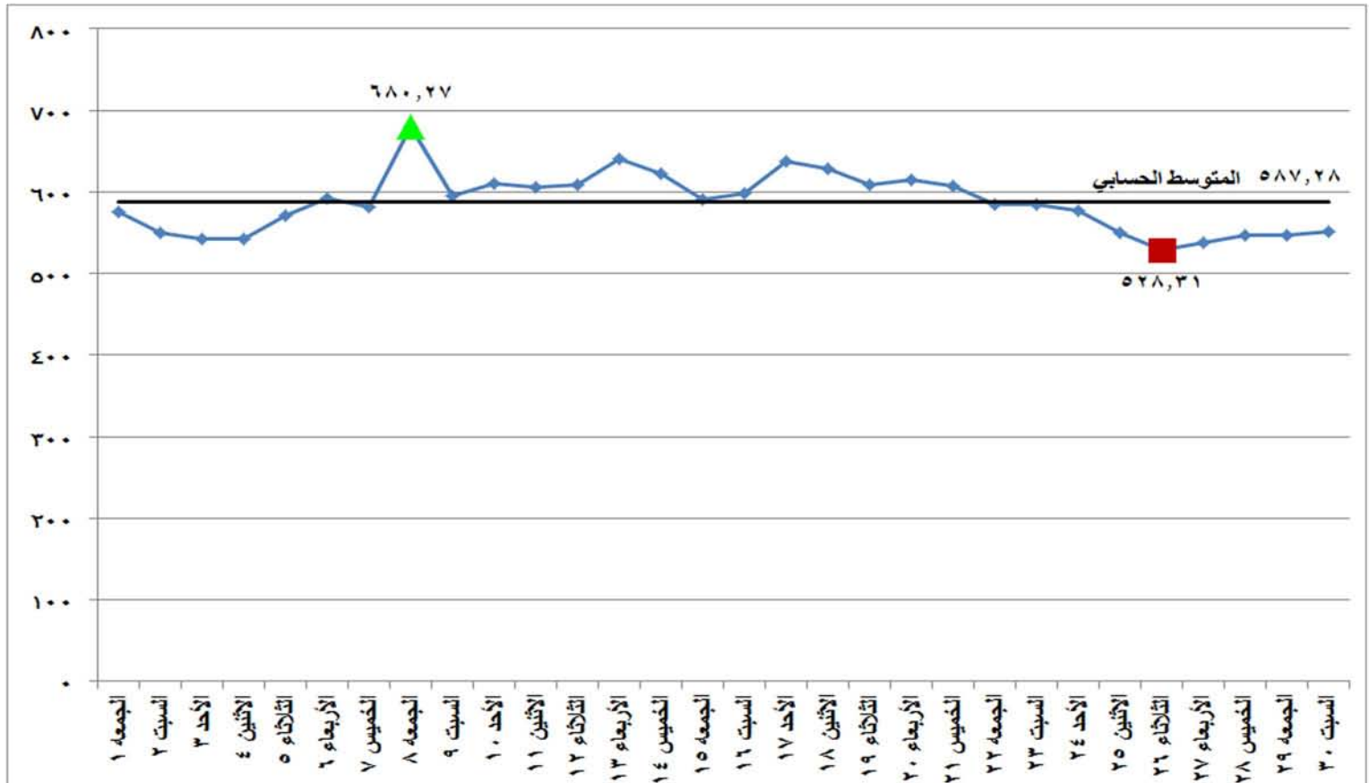
شكل (١٤) معامل انبعاثات غاز ثاني اكسيد الكربون المكافئ على مدى شهر سبتمبر ٢٠١٧
