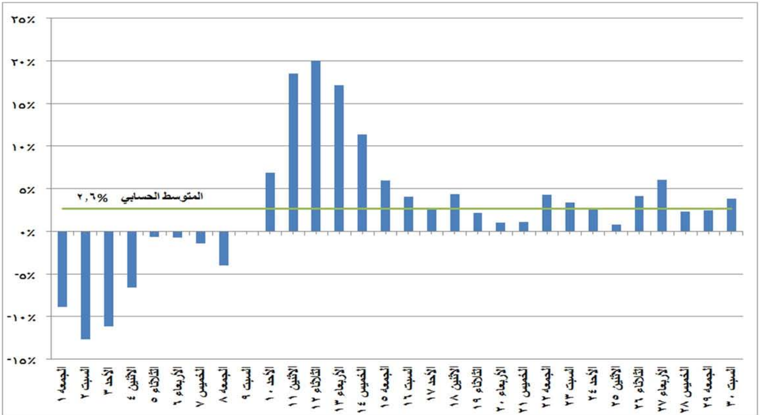
شكل (٩) النسب المئوية للتغير في الحمل الاقصى خلال شهر سبتمبر ٢٠١٧ مقارنة باليوم المماثل من العام الماضي
