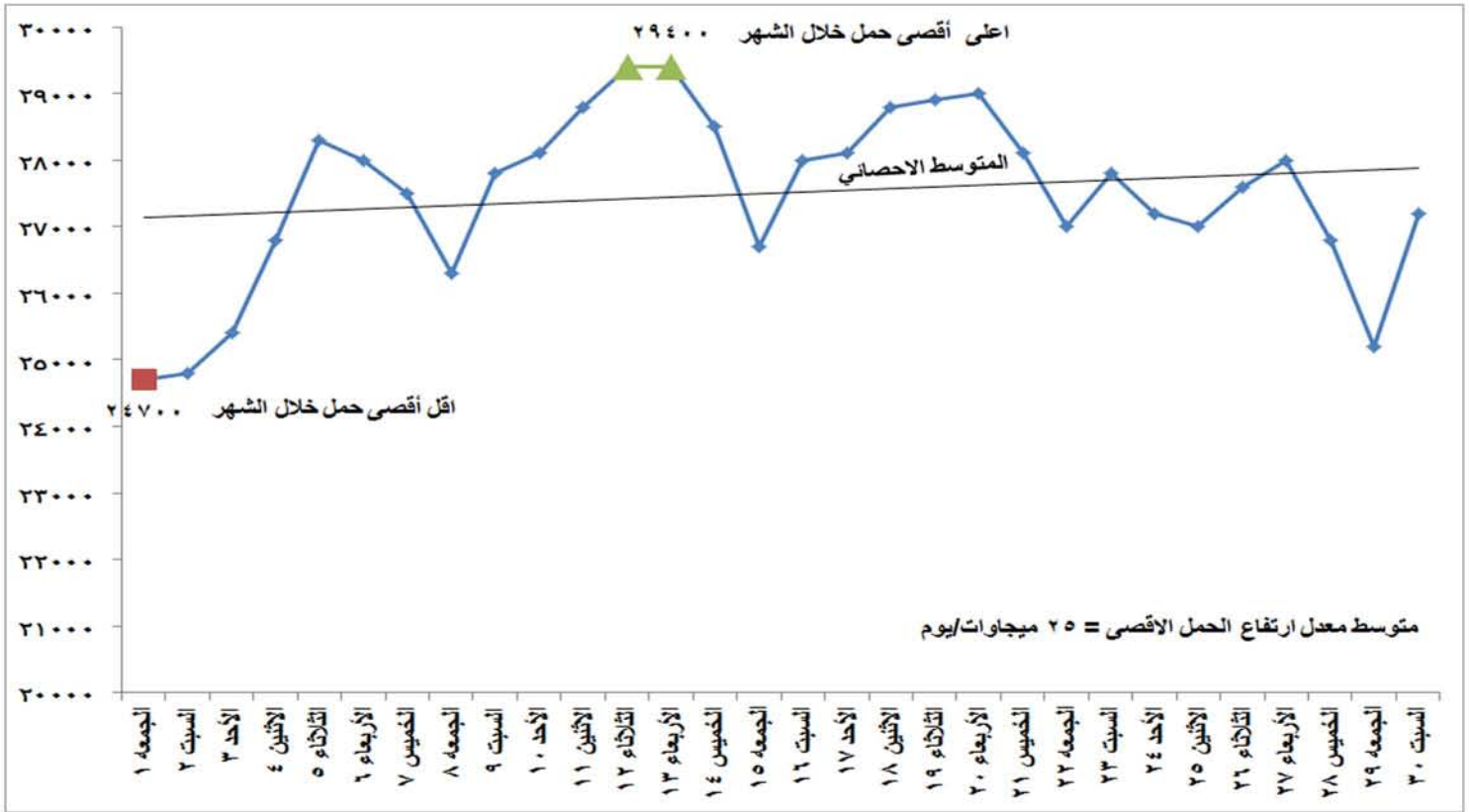
شكل (١) تطور الحمل الاقصى اليومي خلال شهر سبتمبر ٢٠١٧
