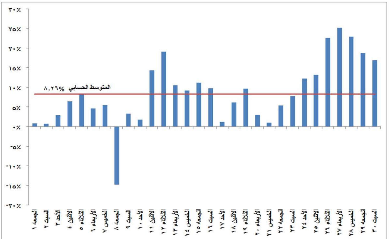
شكل (١٨) نسب التغيير في استخدام الغاز الطبيعي في إنتاج الطاقة الكهربائية خلال شهر سبتمبر ٢٠١٧ مقارنة بالشهر المماثل من العام السابق
