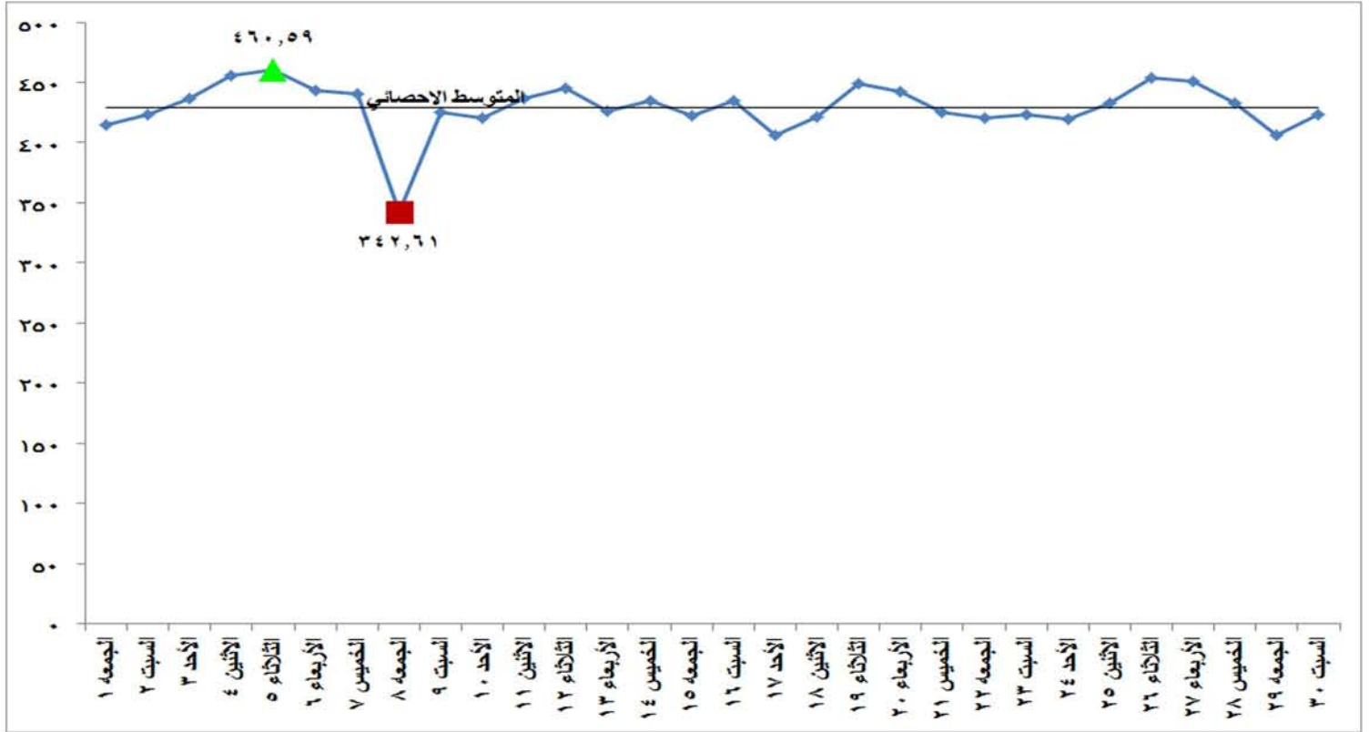
شكل (١٧) الطاقة الكهربائية المنتجة من الغاز الطبيعي خلال شهر سبتمبر ٢٠١٧
