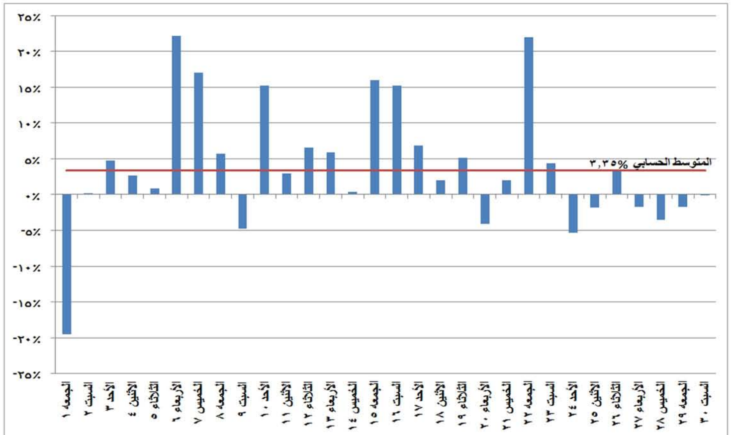
شكل (٢٤) نسب التغير في استخدام المصادر المائية في إنتاج الطاقة الكهربائية خلال شهر سبتمبر ٢٠١٧ مقارنة بالشهر المماثل من العام السابق
