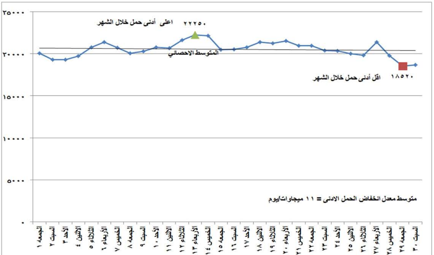
شكل (٢) تطور الحمل الادنى اليومي خلال شهر سبتمبر ٢٠١٧
