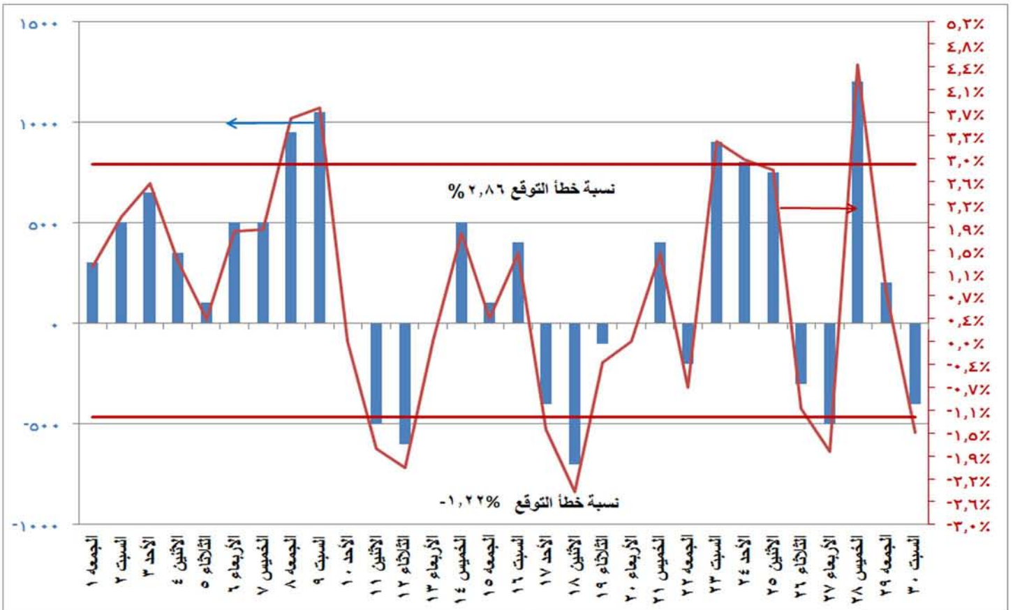
شكل (١٠) الفرق بين الحمل الأقصى المتوقع والمسجل فعليا ونسبة الفرق إلى الحمل المسجل فعليا خلال شهر سبتمبر ٢٠١٧
