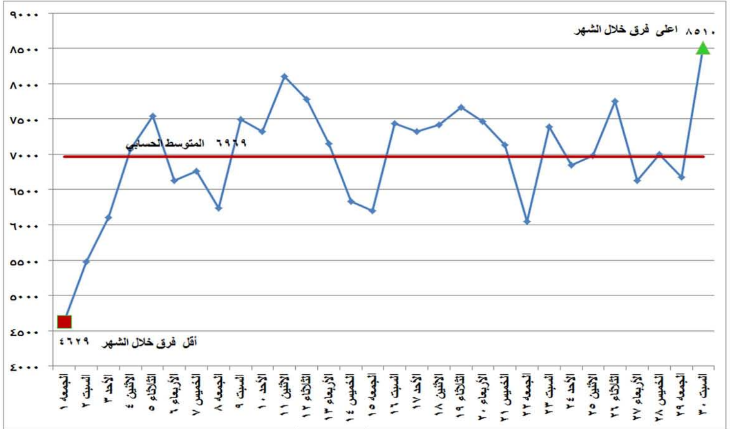
شكل (٣) الفرق بين أقصى وأدنى حمل خلال شهر سبتمبر ٢٠١٧
