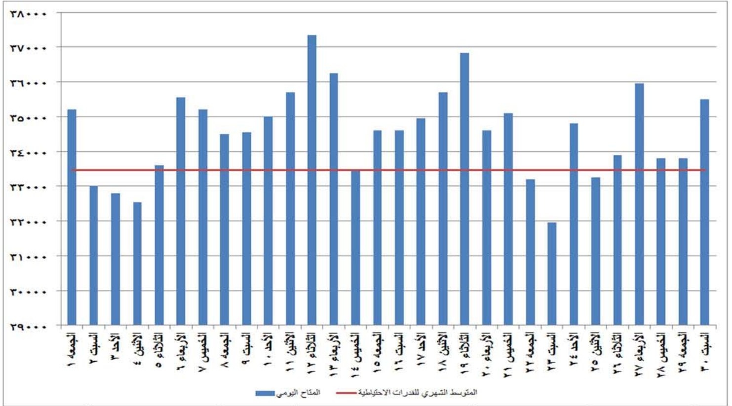
شكل (٢٧) القدرات المتاحة يوميا والمتوسط الشهري للقدرة الاحتياطية خلال شهر سبتمبر ٢٠١٧
