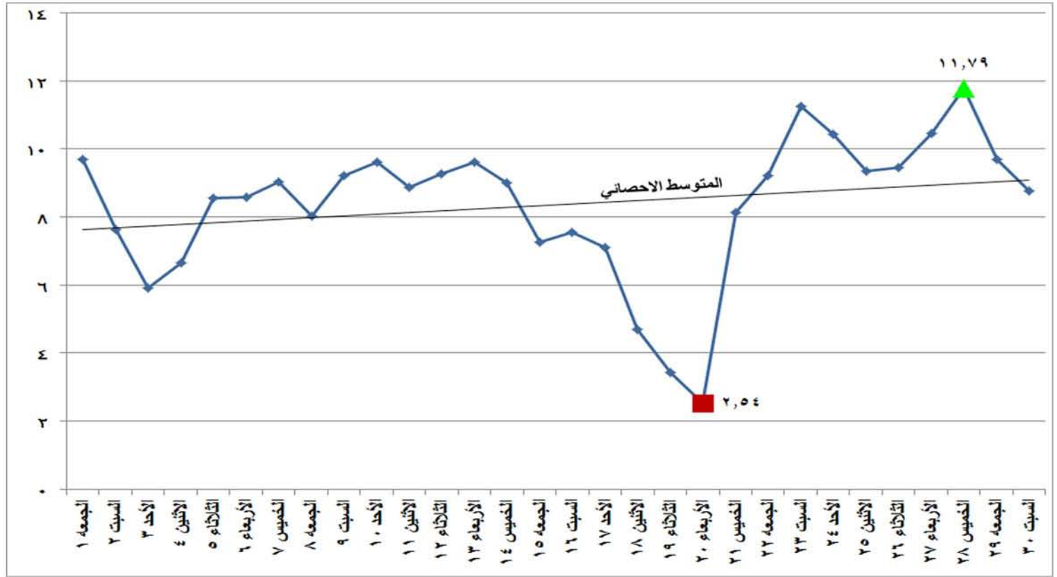
شكل (٢٥) الطاقة الكهربائية المنتجة من الرياح والشمس خلال شهر سبتمبر ٢٠١٧
